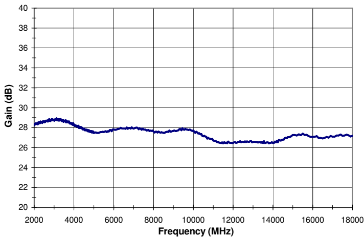
S21
